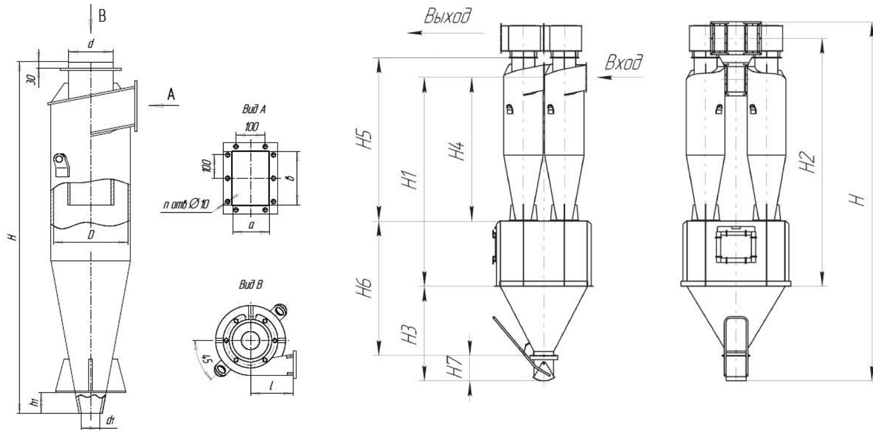
Входной и выходной фланцы
